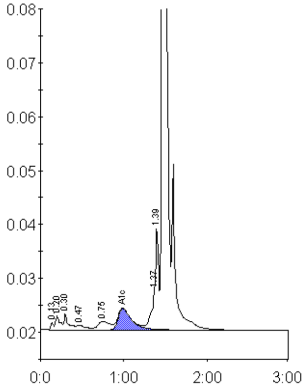
Peak table - ID: 60001249
